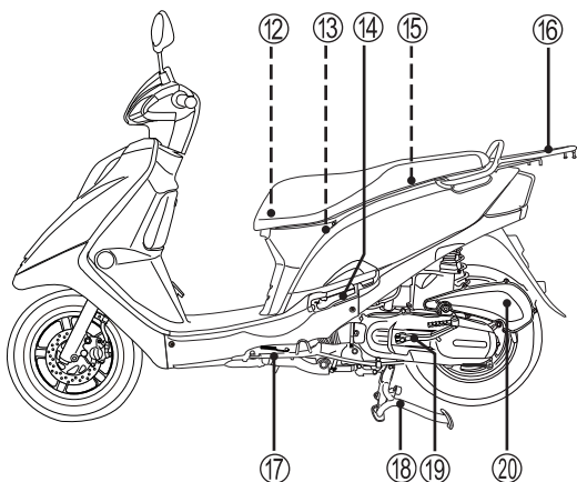
QS125T-6 NG/NS( 脚制动型 )
